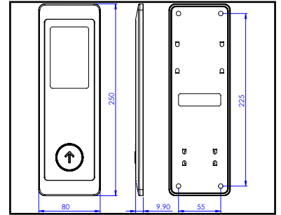
dimensions 32
